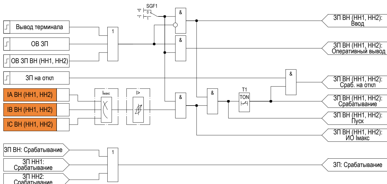
Рисунок 2.14 – Функциональная схема «ЗП»
